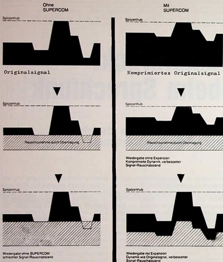
Bild 2. Funktionsweise des Rausch- und Störunterdrückungssystems Supercom
