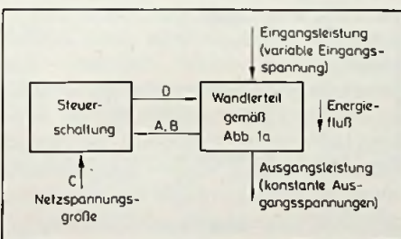
Bild 2. Signallauf des Wandlers
