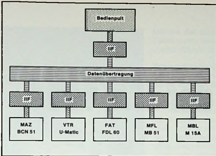
Bild 1. Entscheidend für das elektronische Schnittsystem für unterschiedliche Informationsträger ist das Intelligente Interface IFF
