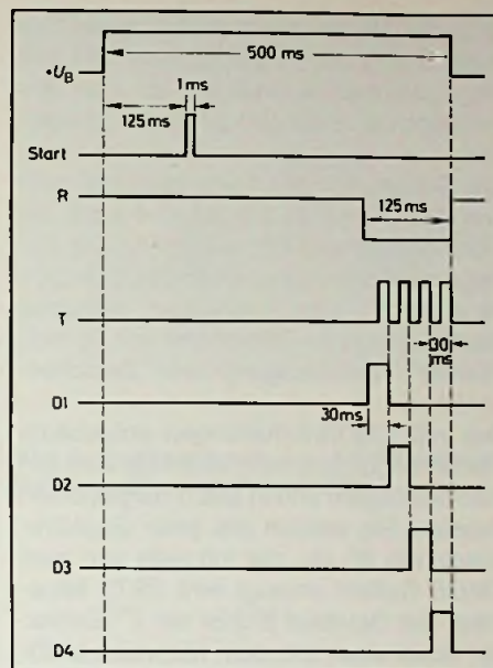
Bild 5. Impulsplan der Takterzeugung
