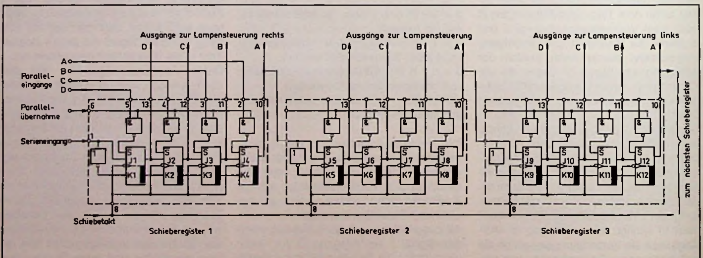
Bild 3. Zusammenwirken integrierter Schieberegister in Laufflichtsteuerungen
