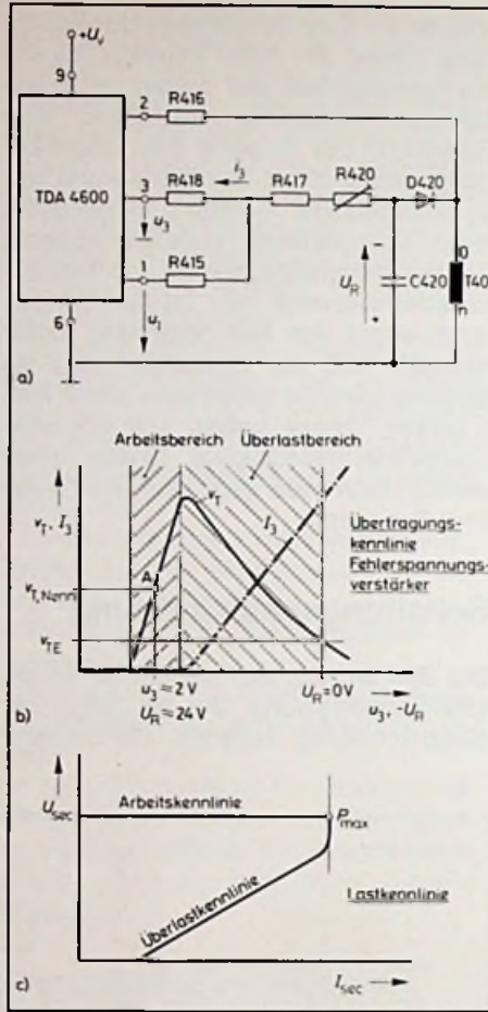
Bild 4. (links) a) Fehlerspannungsverstärker (Stift 3), Nullspannungsindikator (Stift 2) und Referenzspannungsquelle (Stift 1); b) Übertragungsfunktion des Fehlerspannungsverstärkers. Der Funktionsverlauf im Überlastbereich wird durch den Strom I_3 bestimmt; c) Lastkennlinie. Der rückläufige Verlauf der Überlastkennlinie schützt das Gesamtsystem vor Zerstörung
