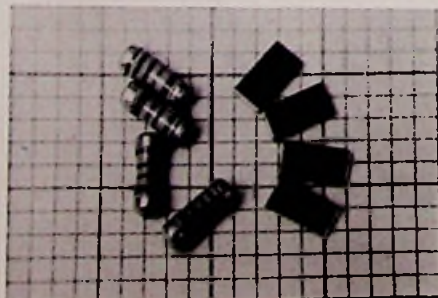
Bild 5. Widerstände für modernste Bestückungsverfahren; rechts: Chip-Widerstände, links: MELF-Widerstände
