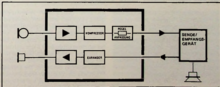
Bild 1. Blockschaltdiagramm des Rausch- und Störunterdrückungssystems Supercom von AEG-Telefunken
