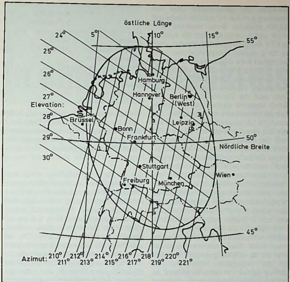
Bild 2. Elevations- und Azimutwinkel abhängig vom Wohnort. Die Werte sind nur gültig zum Ausrichten der Empfangsantenne auf die Orbitposition – 19°. Je größer der Elevationswinkel ist, desto weniger sind Abschattungen zu befürchten (Hirschmann)
