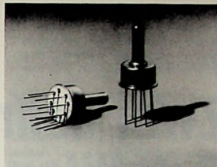
Bild 9. Drucksensoren im TO-8-ähnlichen Gehäuse (Siemens-Pressbild)
